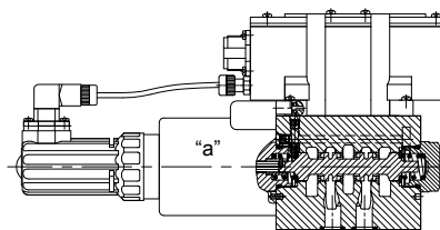
型号 4WREE 10...A-2X/...
