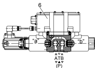
型号 4WREE 6...-2X/...
