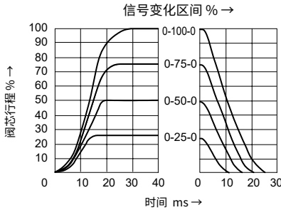
输入信号为阶跃信号时阀的过渡性能
