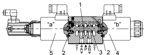
型号 4WRE 10...-2X/...
