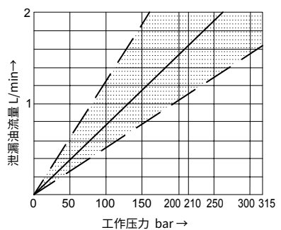
型号 4WREE10 V75
