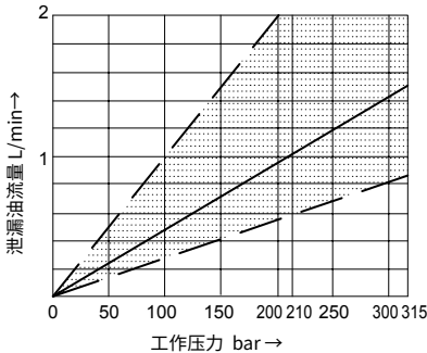
型号 4WREE6 V32
